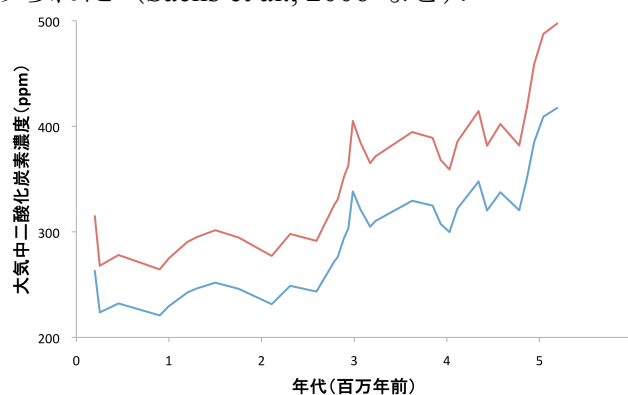
図 2. アルケノンと有孔虫の炭素同位体組成から推定された過去 500 万年間の大気二酸化炭素濃度 (Seki et al., 2010). 赤: 上限値, 青: 下限値.
